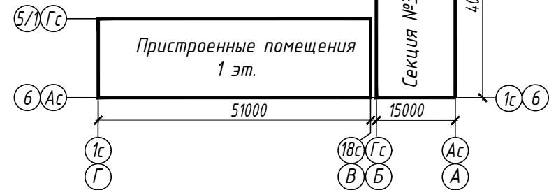
Схема блокировки
